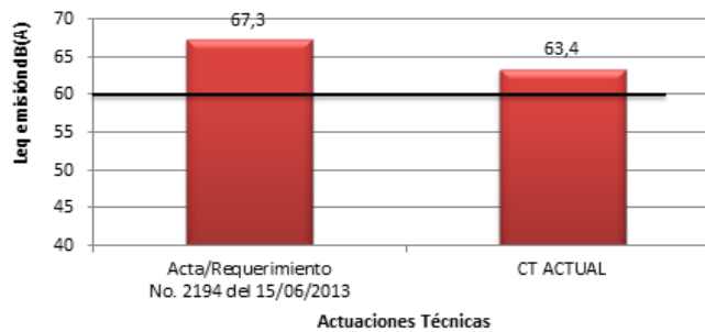
Gráfica 1. Histórico de ruido
